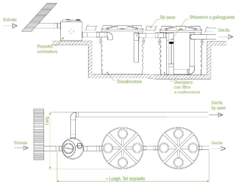
SCHEMA DI IMPIANTO DI PRIMA PIOGGIA CON SCARICO SU PUBBLICA FOGNATURA
