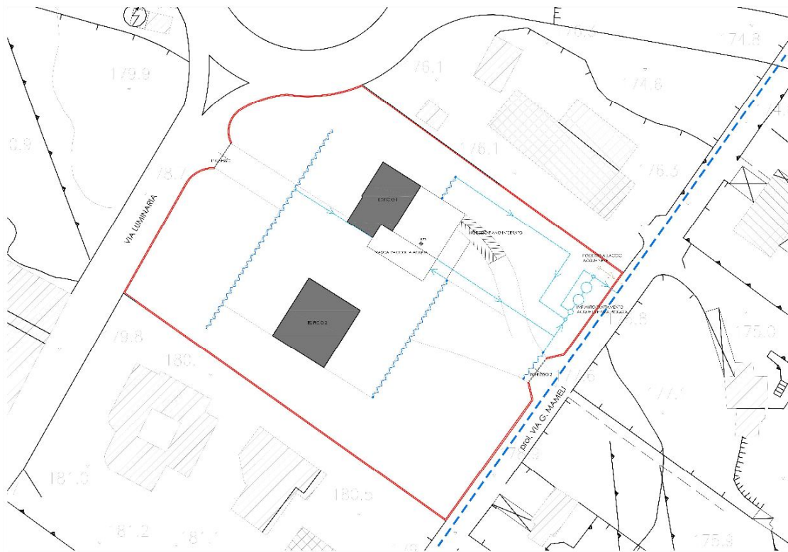
SCHEMA DI IMPIANTO DI PRIMA PIOGGIA CON SCARICO SU PUBBLICA FOGNATURA
